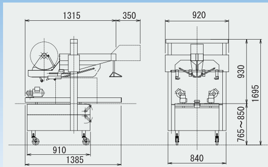
■外形図
