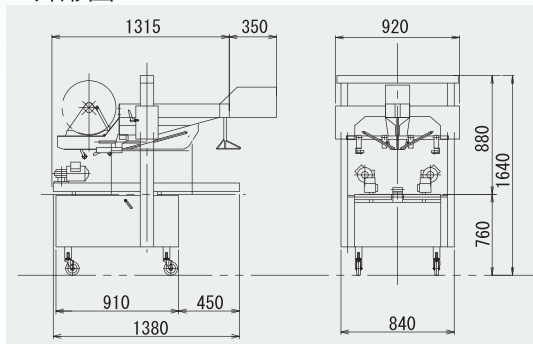
■外形図
